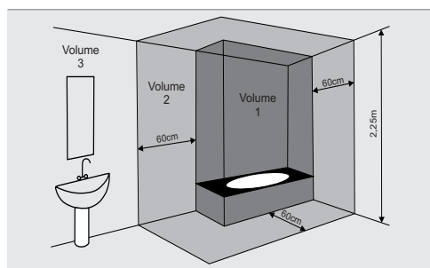
Abb.1: Sicherheitsabstände
