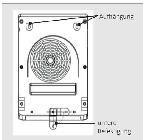
Abb.4: Anbringung
