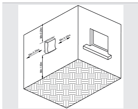
Abb.2: Montage Maße
