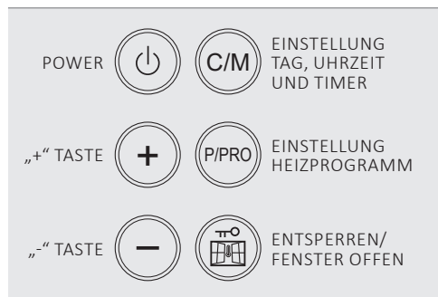
Abb.5b: Bedieneinheit
