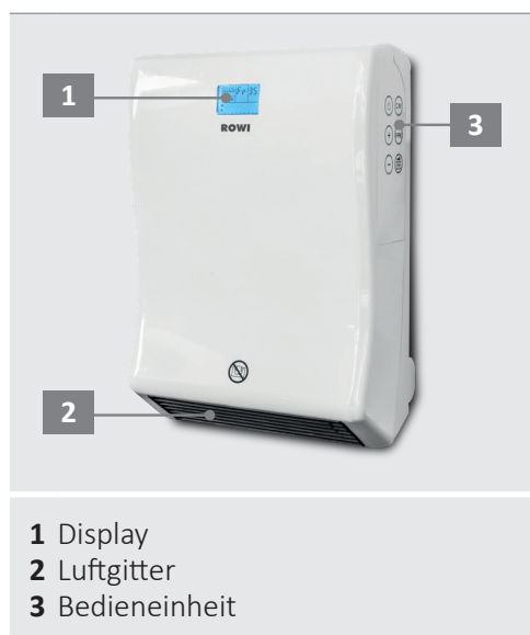
Abb.5a: Geräteübersicht
