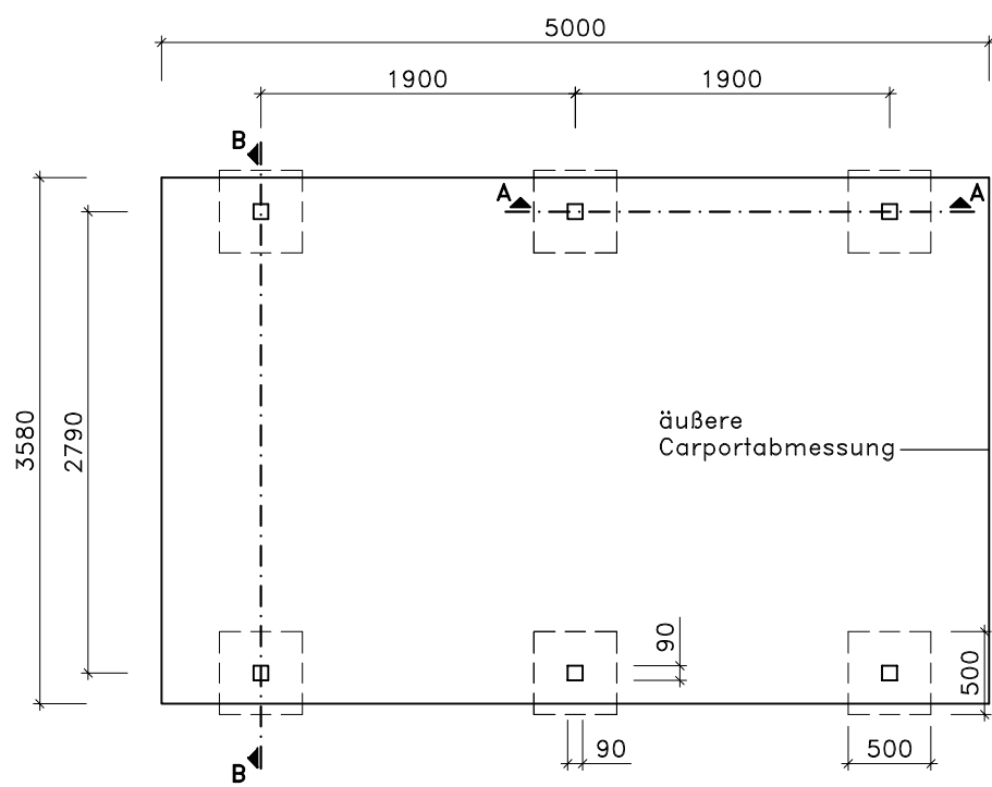
Grundriß
