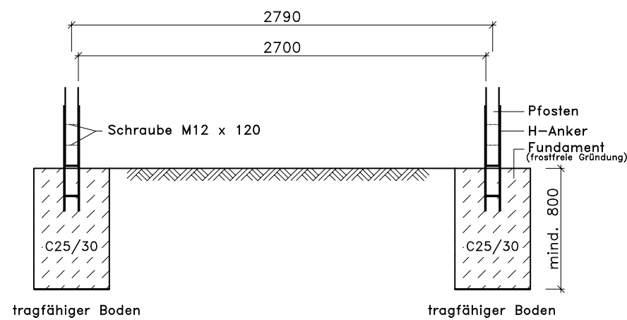
Schnitt B-B
