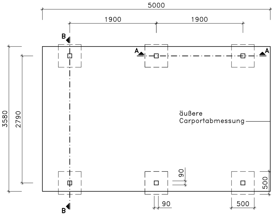
Grundriß
