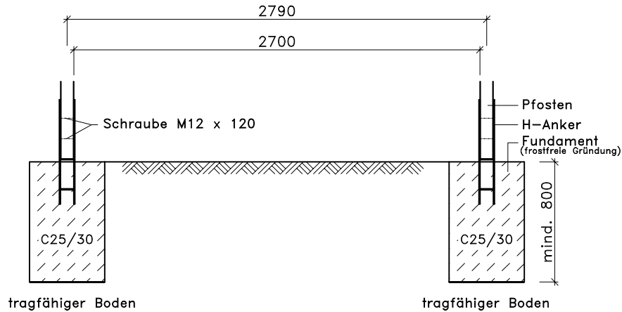
Schnitt B-B
