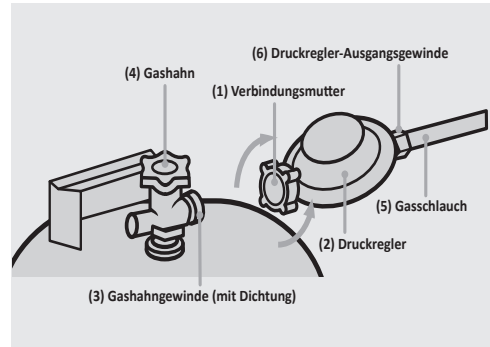
Abb.2: Montage des Druckreglers
