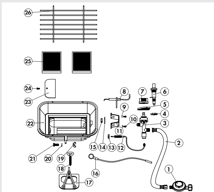
Abb. 4: Explosionszeichnung
