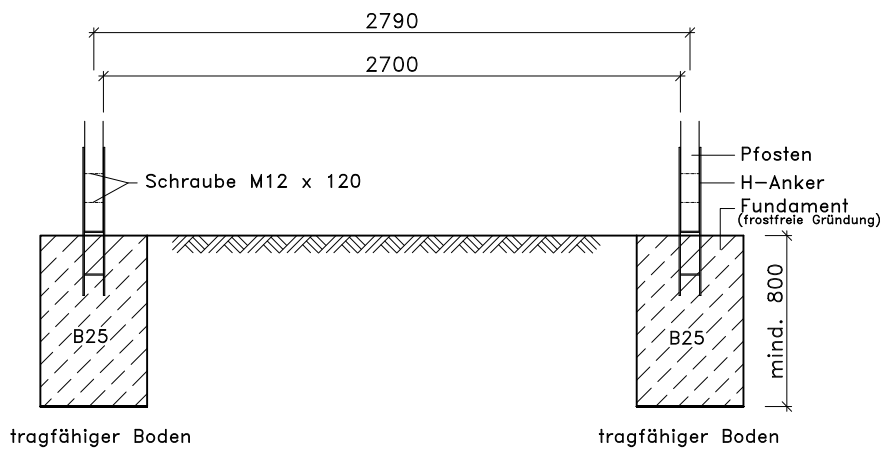
Schnitt B-B
