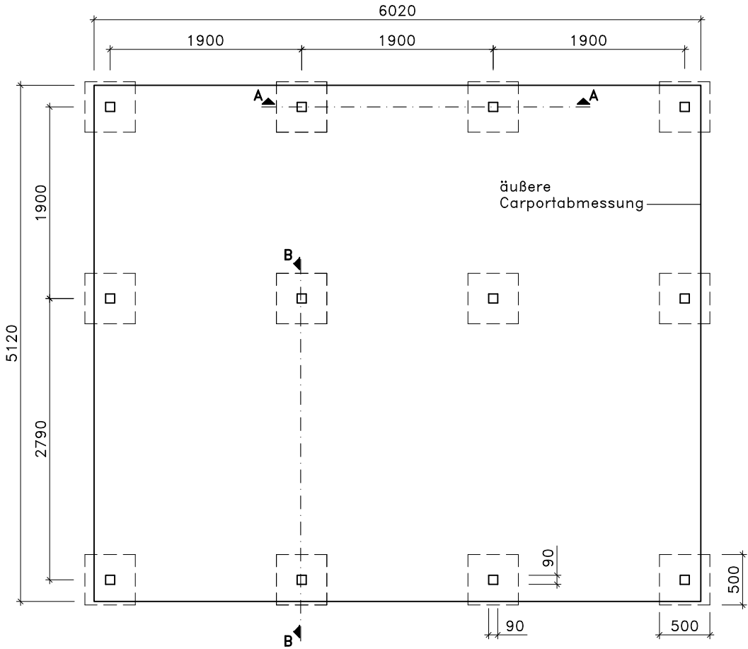
Grundriß
