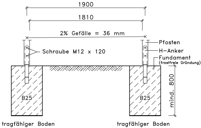
Schnitt A-A
