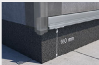
Befestigung des Starterprofils
