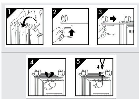
Abb.1: Montage Räder
